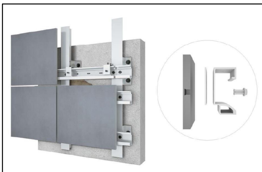
شکل شماره ۲- شماتیک اجرای سرامیک پرسلانی خشک
