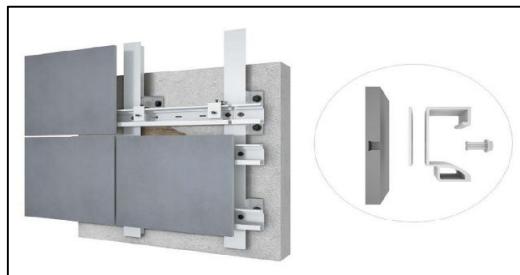
شکل شماره ۲- شماتیک اجرای سرامیک پرسلانی خشک
